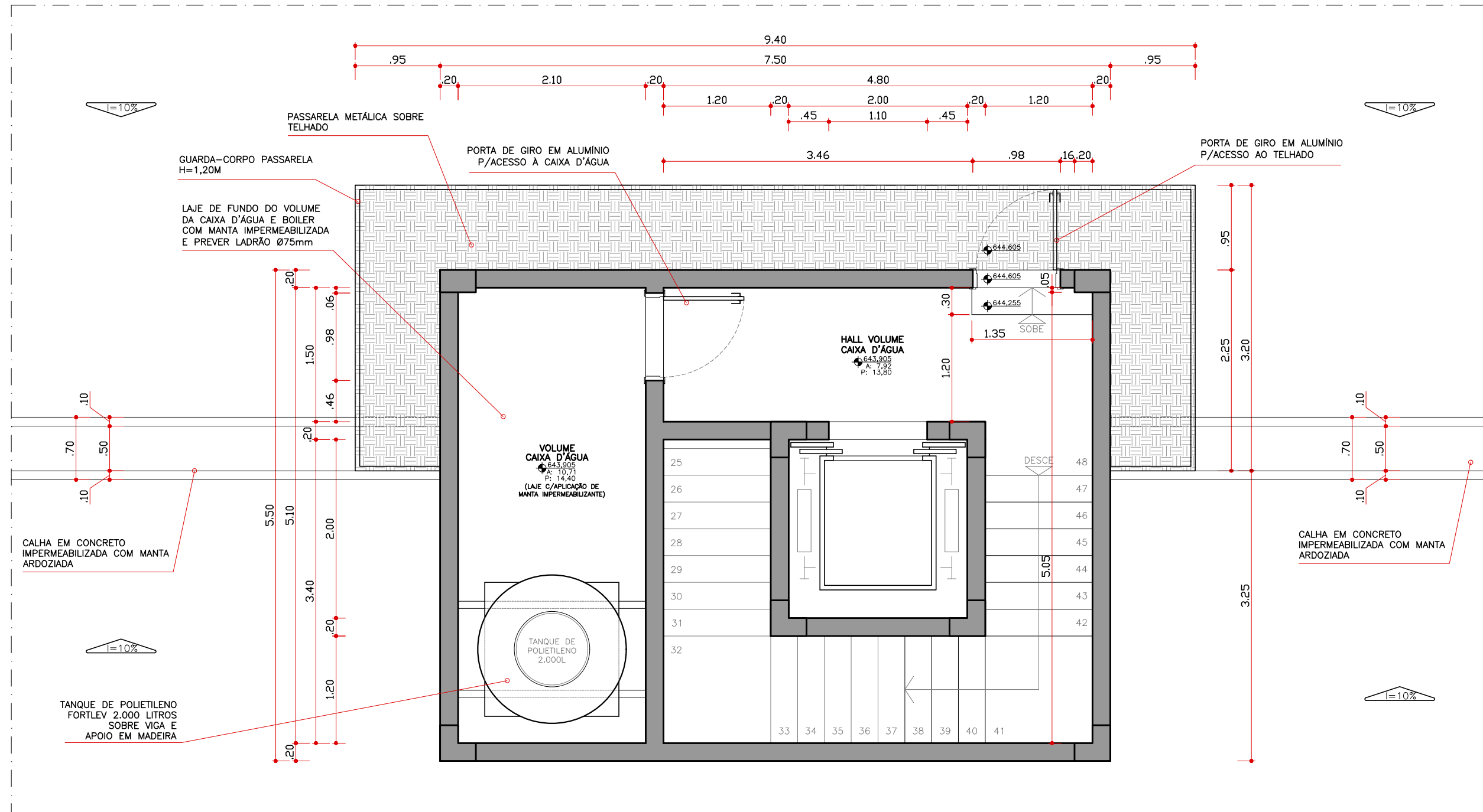
PLANTA BAIXA - VOLUME CAIXA D'ÁGUA ESC. 1:50
