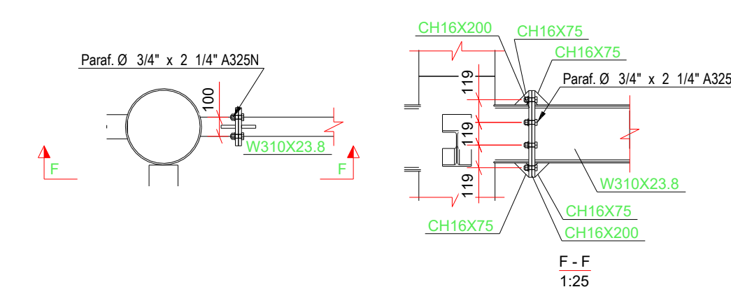
DET. TIPICO W310 NO PILAR
