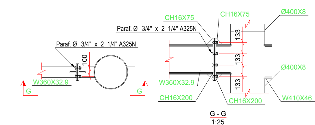
DET. TIPICO W360 NO PILAR
