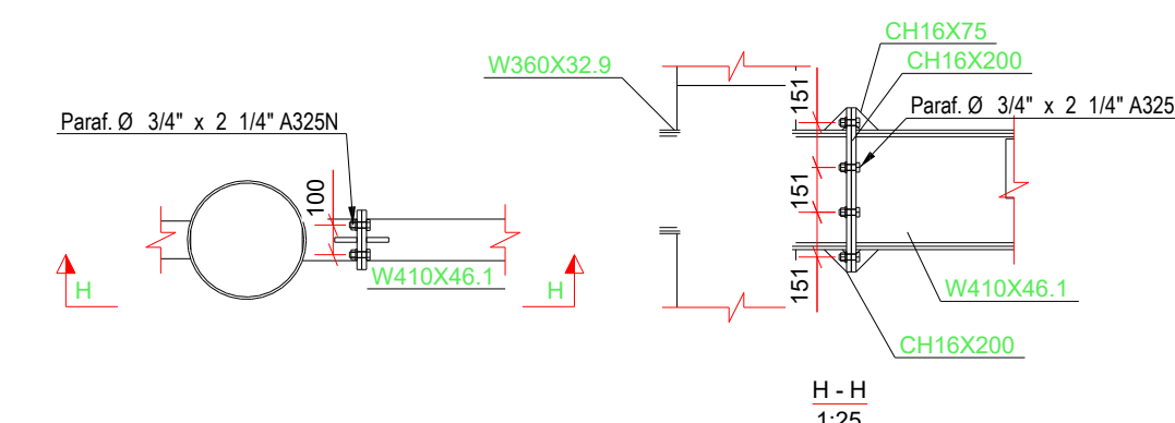
DET. TIPICO W410 NO PILAR
