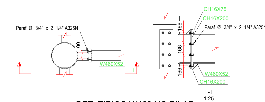
DET. TIPICO W460 NO PILAR
