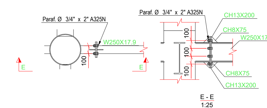
DET. TIPICO W250 NO PILAR
