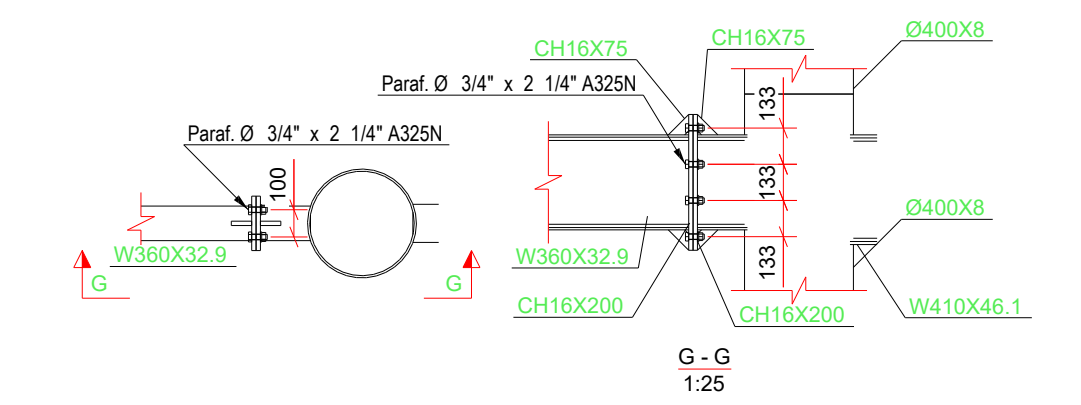
DET. TIPO W360 NO PILAR
