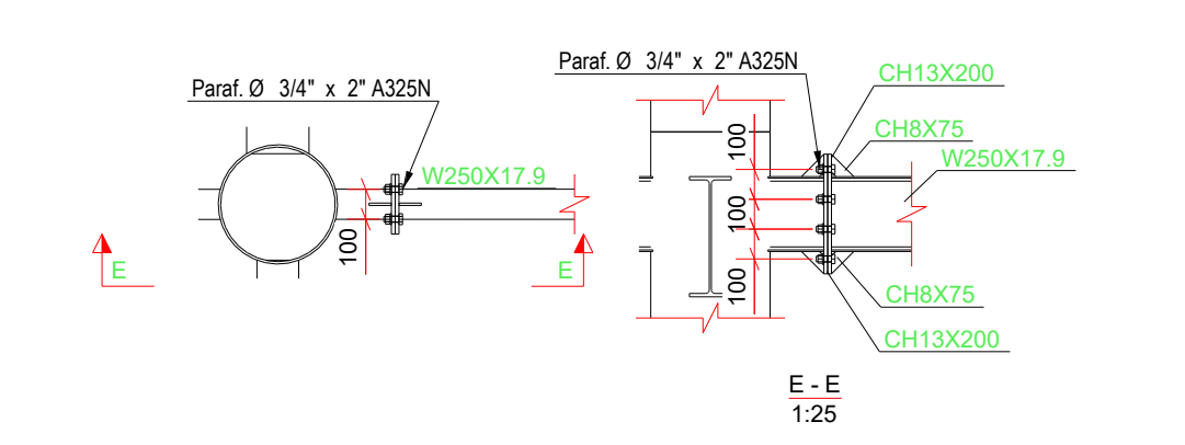
DET. TIPO W250 NO PILAR
