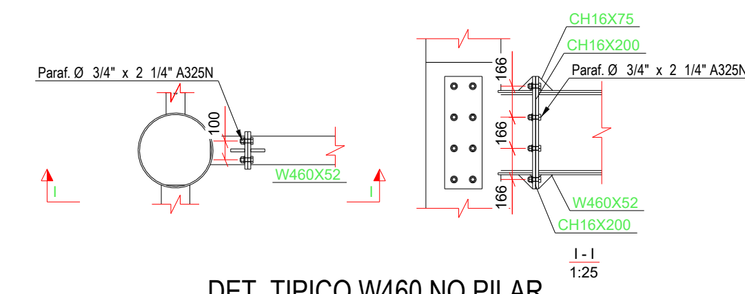
DET. TIPO W460 NO PILAR
