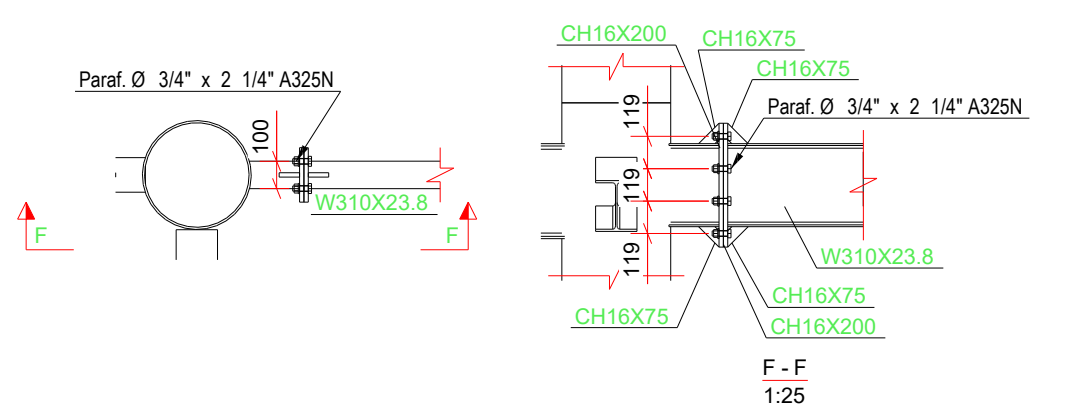
DET. TIPO W310 NO PILAR
