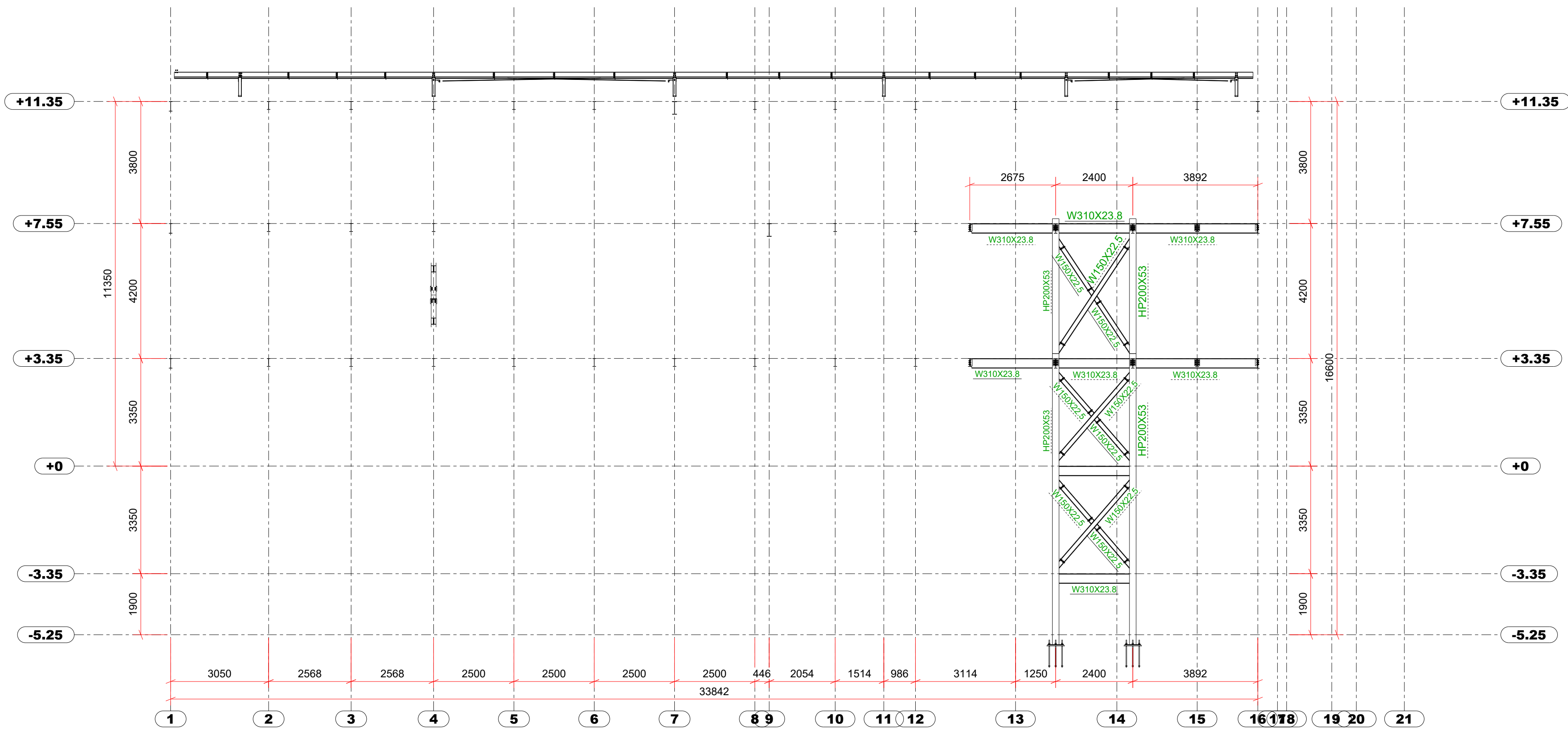
ELEVAÇÃO FILA "E" ESC. 1:100
