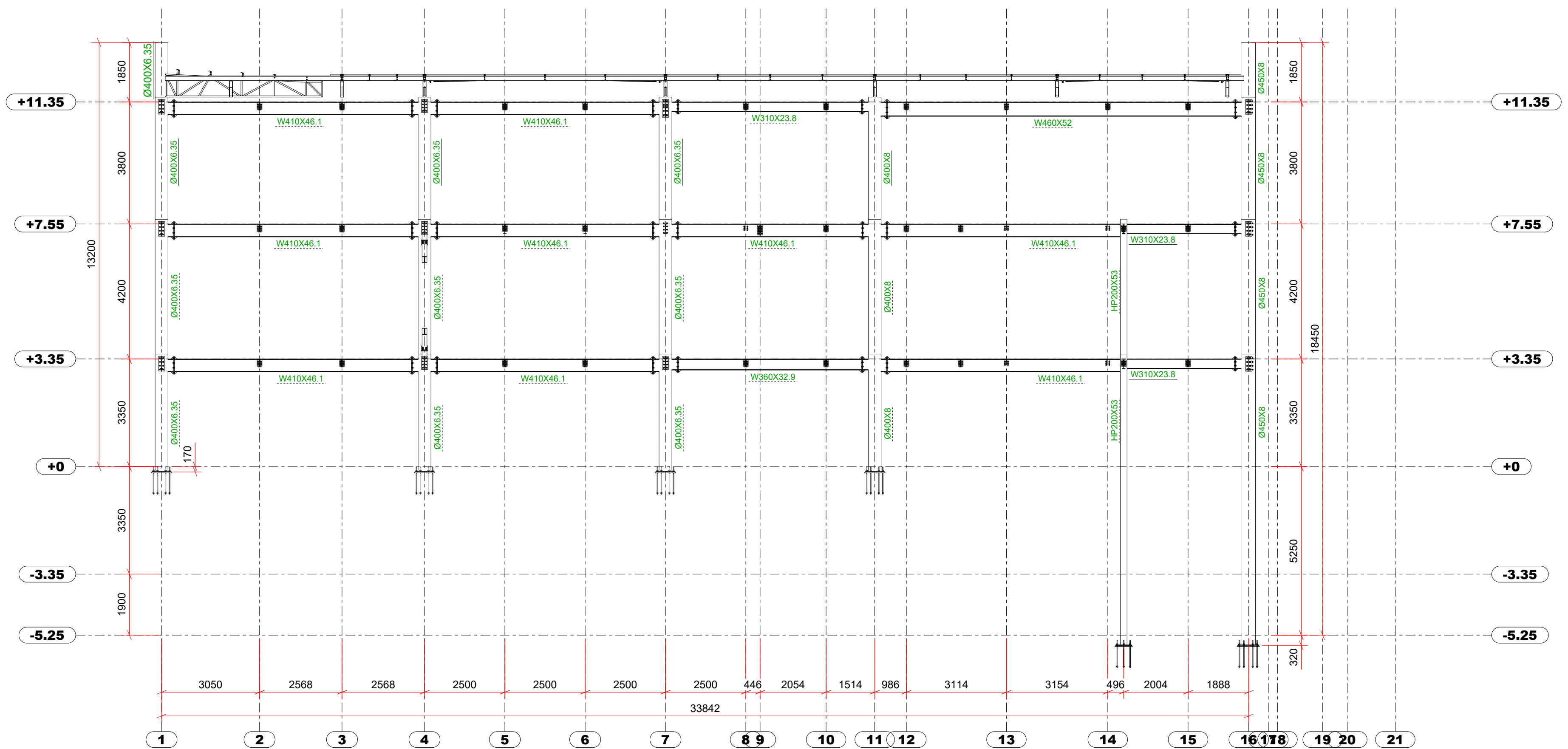
ELEVAÇÃO FILA "F" ESC. 1:100
