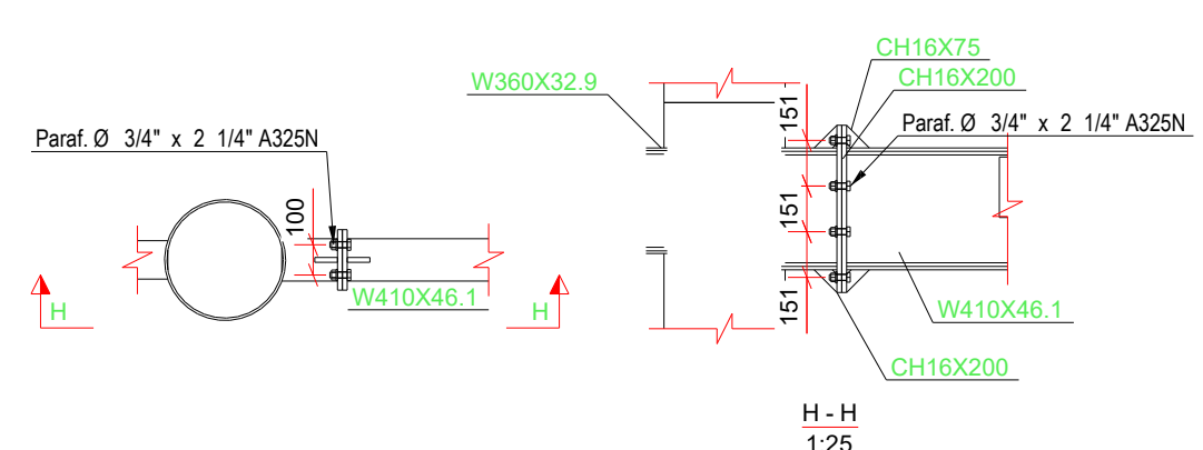
DET. TIPO W410 NO PILAR
