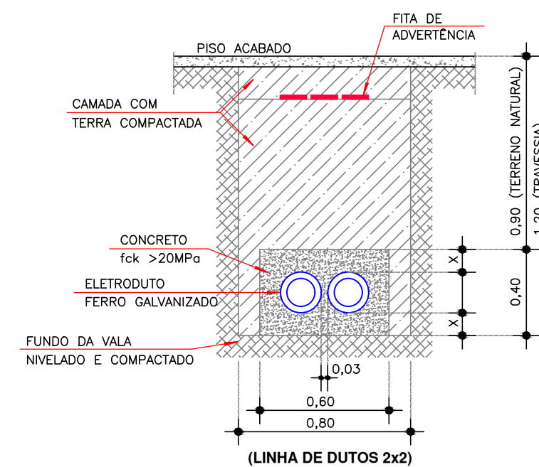
DETALHE BANCO DE DUTOS ENTERRADOS SEM ESCALA
