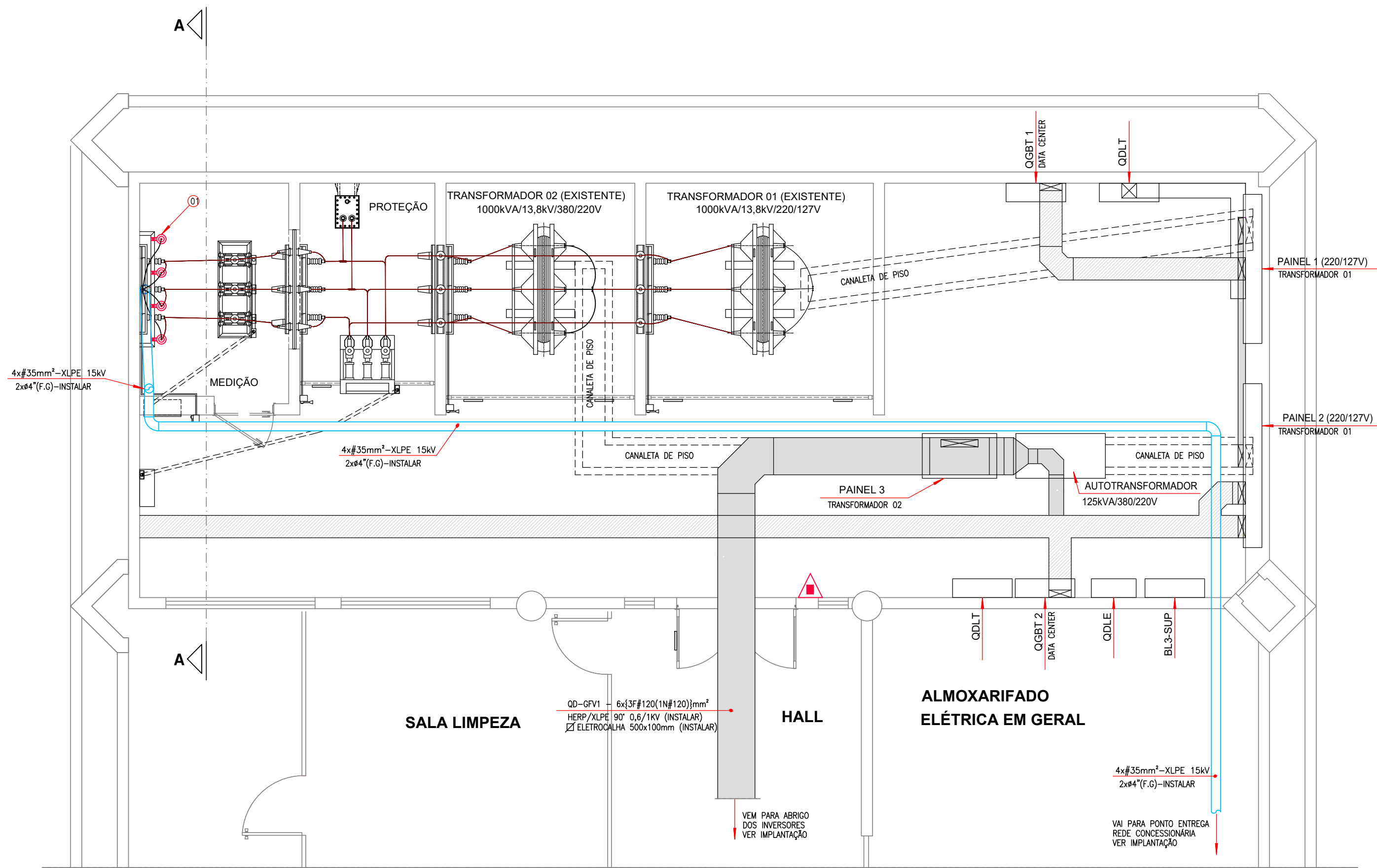
PLANTA BAIXA - SUBESTAÇÃO MEDIÇÃO/PROTEÇÃO E TRANSFORMAÇÃO ESCALA 1:50
