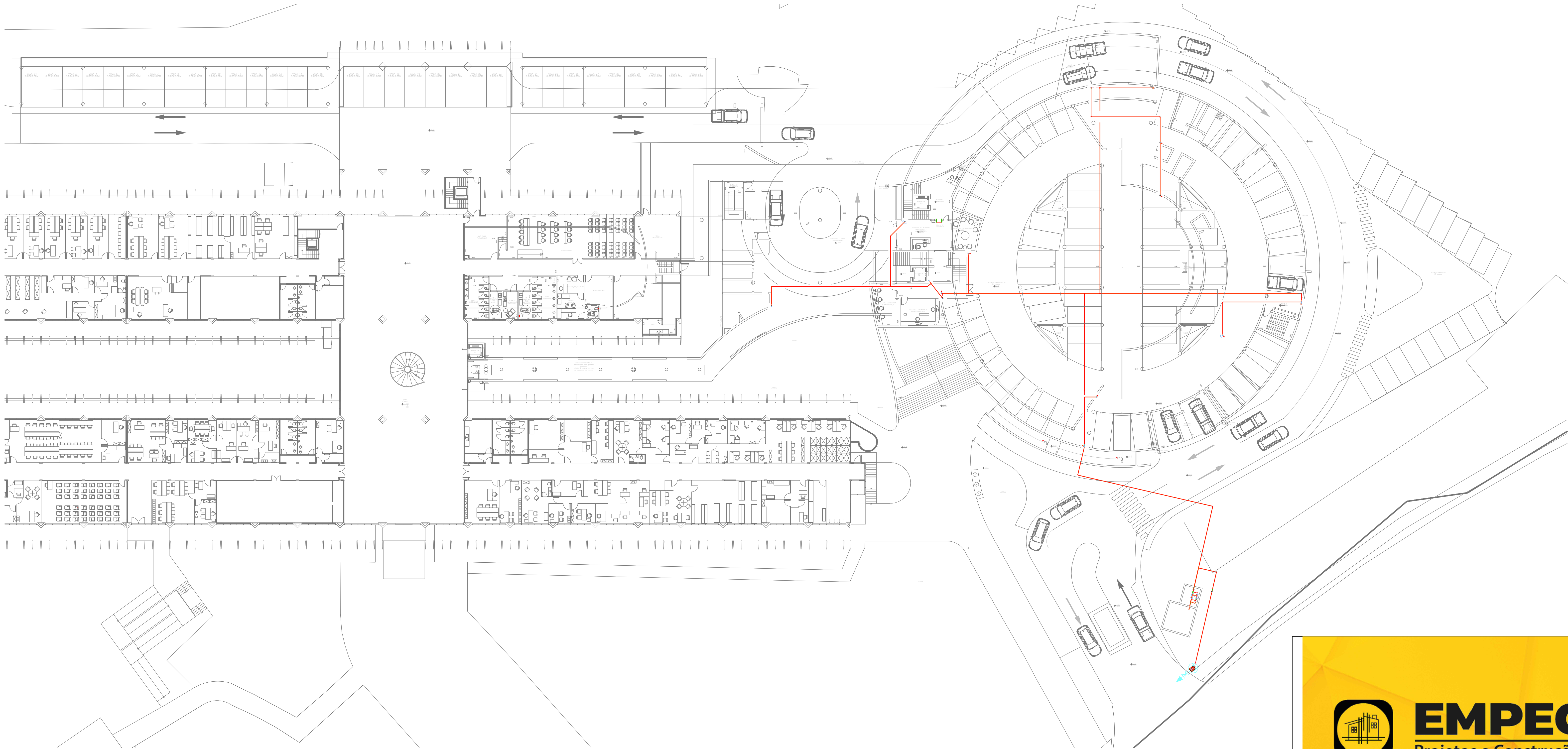
1 00 - Implantação - Caminhamento Hidrante sem escala
