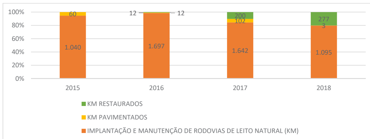
Gráfico 30 - Km de obras concluídas de rodovias estaduais
