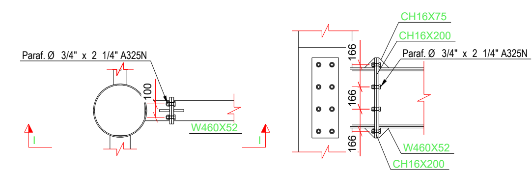
DET. TÍPICO W460 NO PILAR
