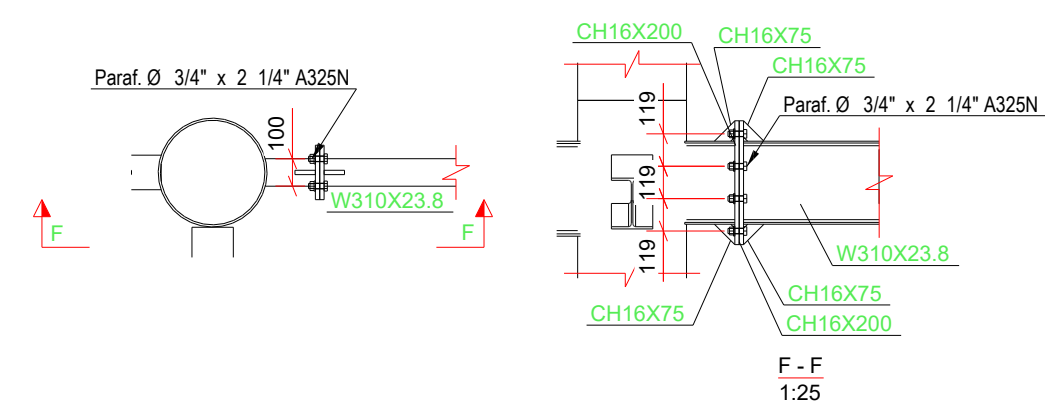
DET. TÍPICO W310 NO PILAR
