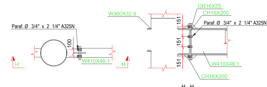
DET. TÍPICO W410 NO PILAR
