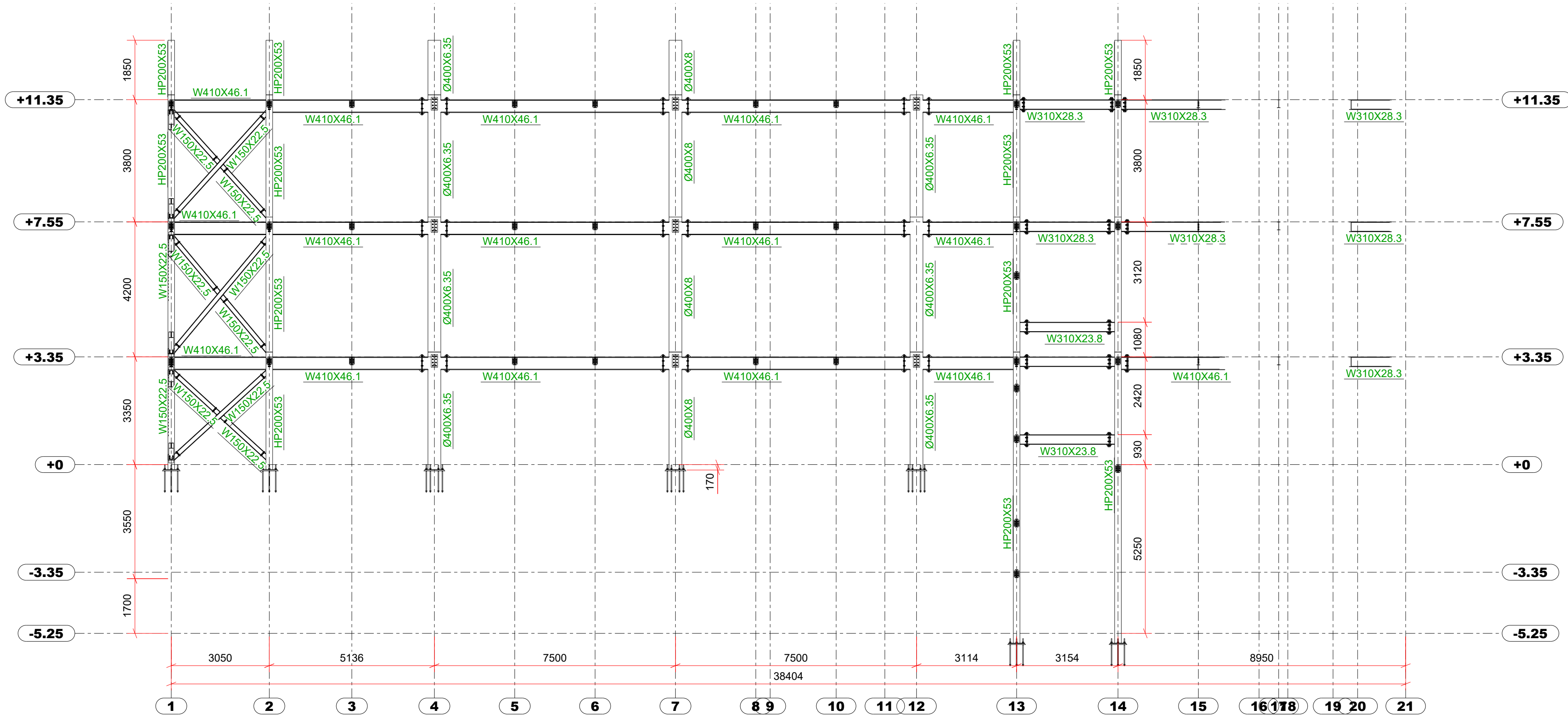
ELEVACÃO FILA "K" ESC. 1:100
