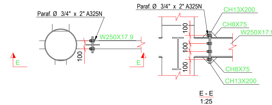
DET. TÍPICO W250 NO PILAR
