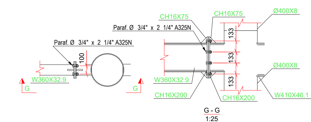
DET. TÍPICO W360 NO PILAR
