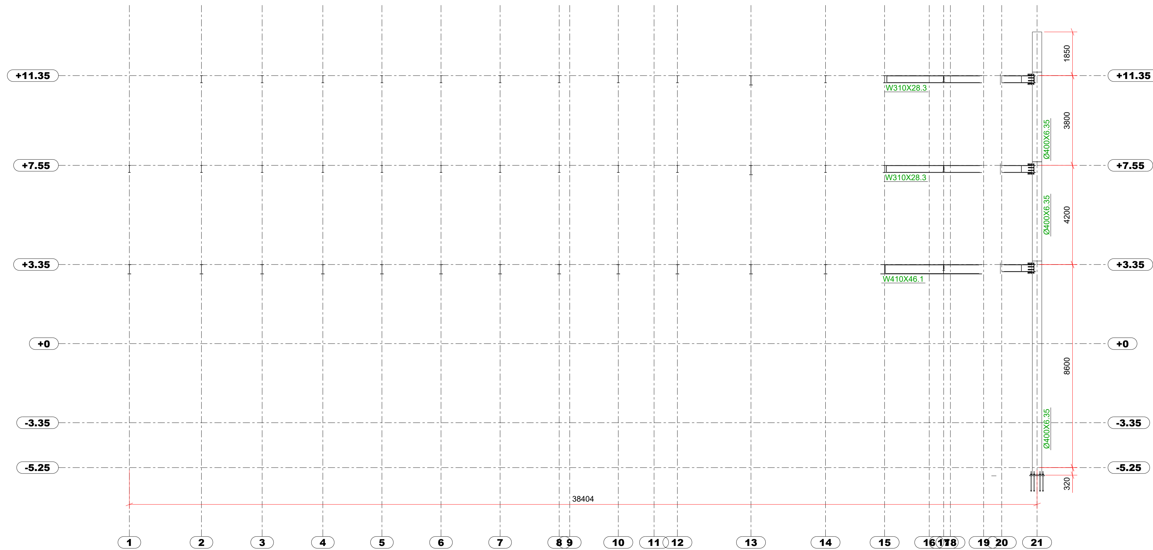
ELEVACÃO FILA "L" ESC. 1:100
