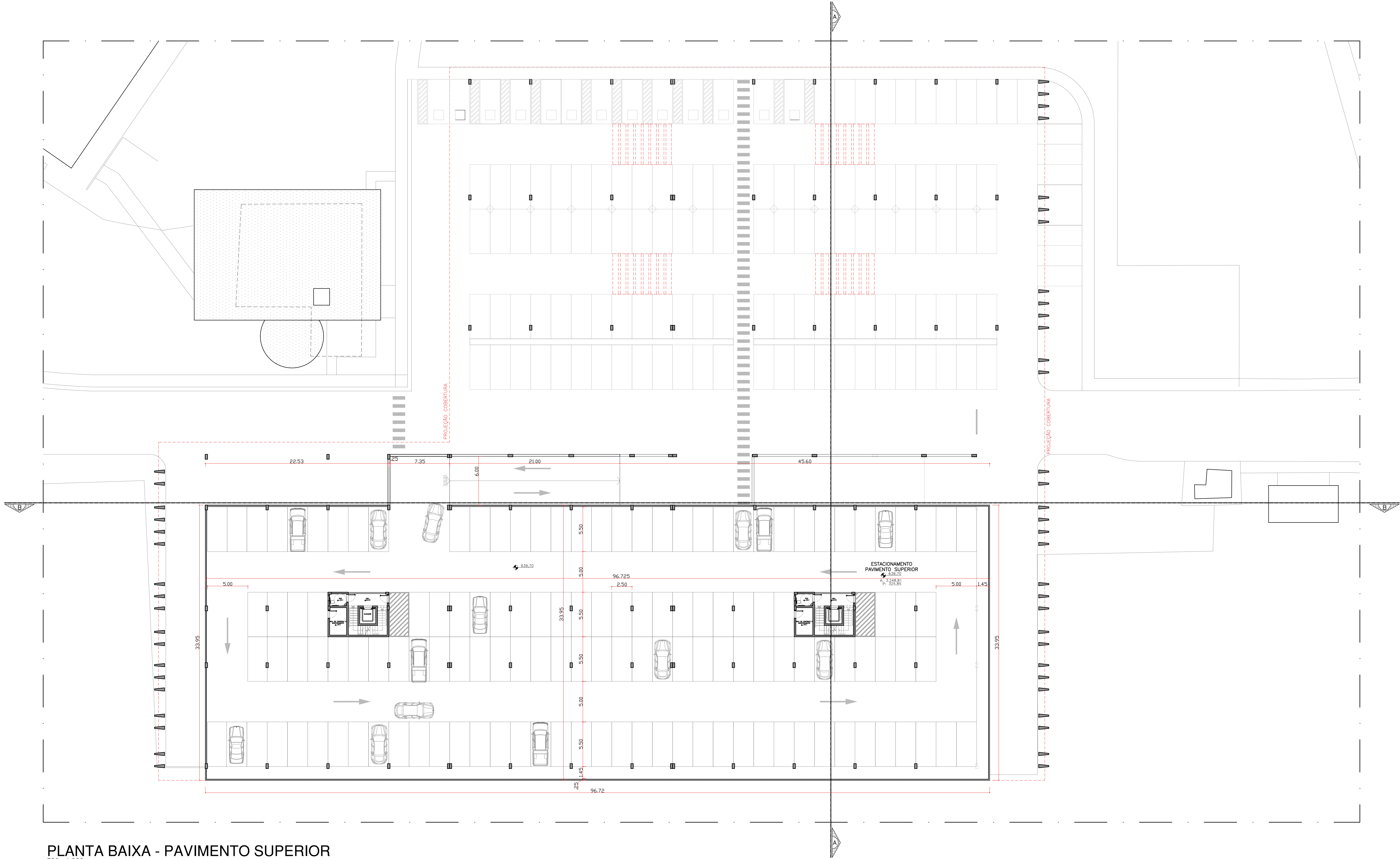
PLANTA BAIXA - PAVIMENTO SUPERIOR
