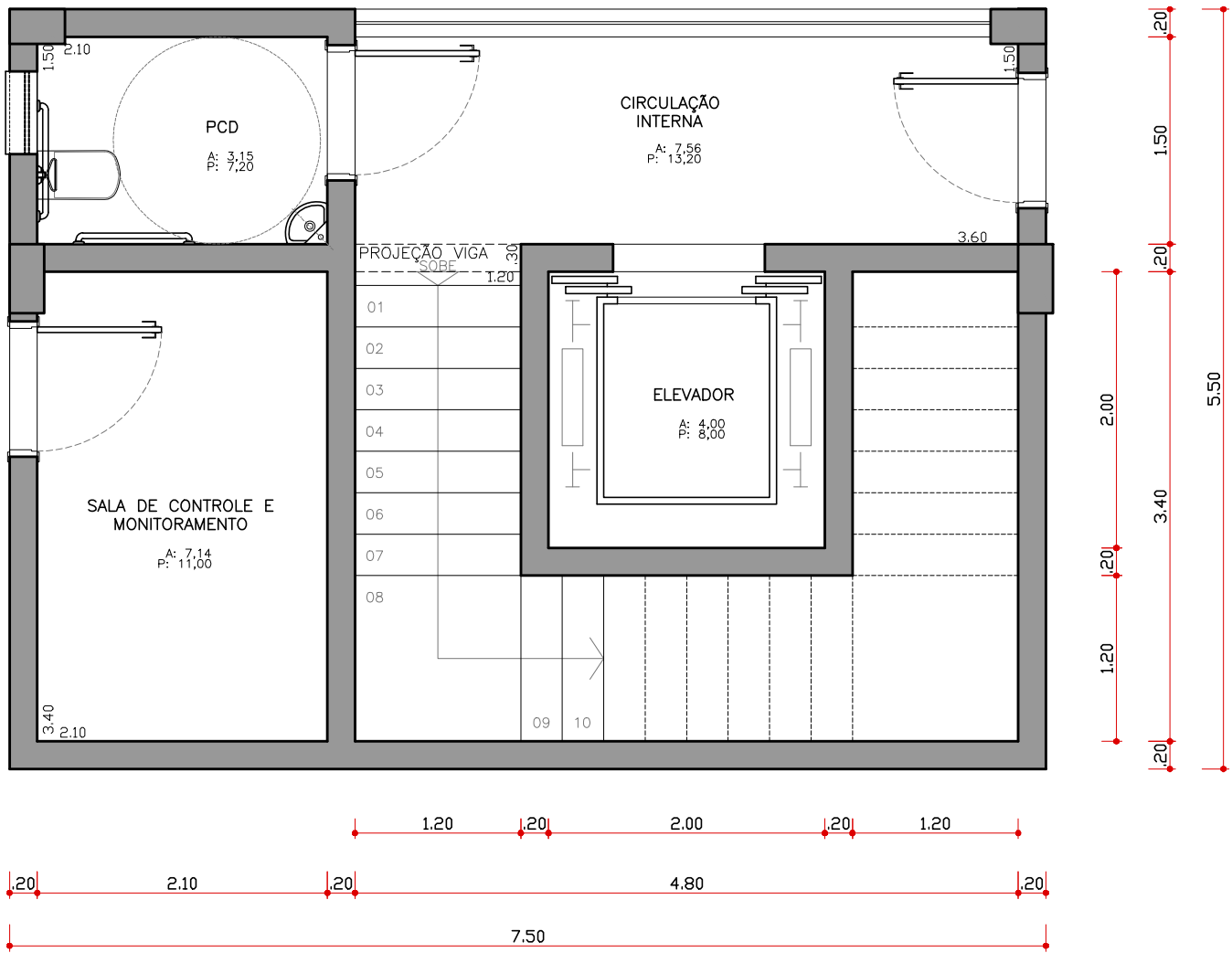
PLANTA BAIXA - BLOCO ESCADA
