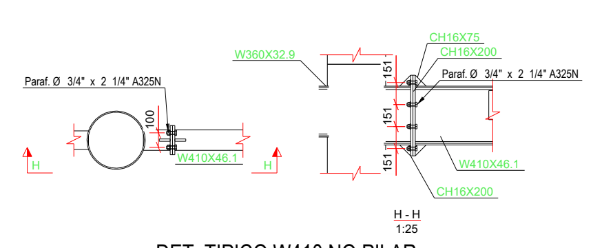
DET. TÍPICO W410 NO PILAR
