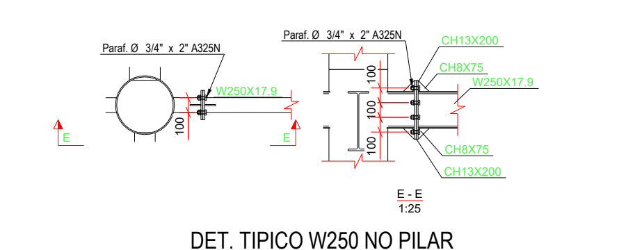
DET. TÍPICO W250 NO PILAR
