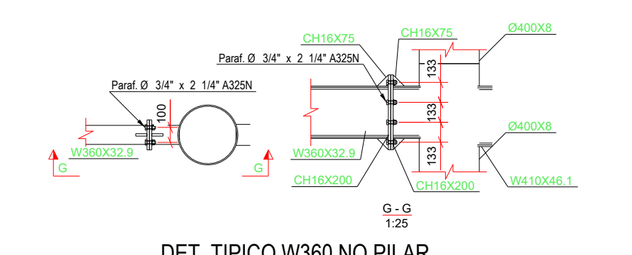
DET. TÍPICO W360 NO PILAR
