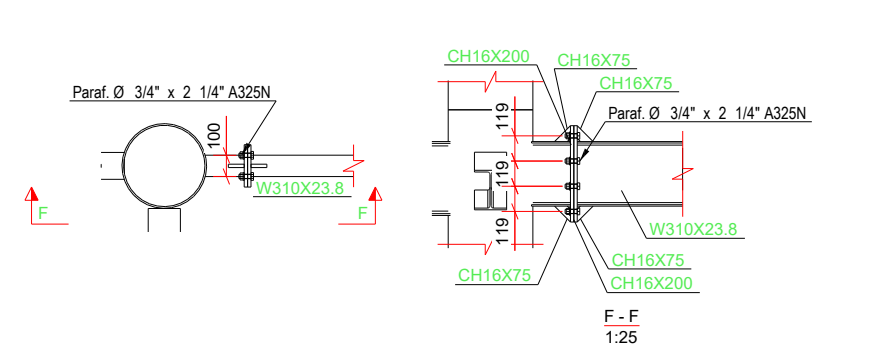
DET. TÍPICO W310 NO PILAR
