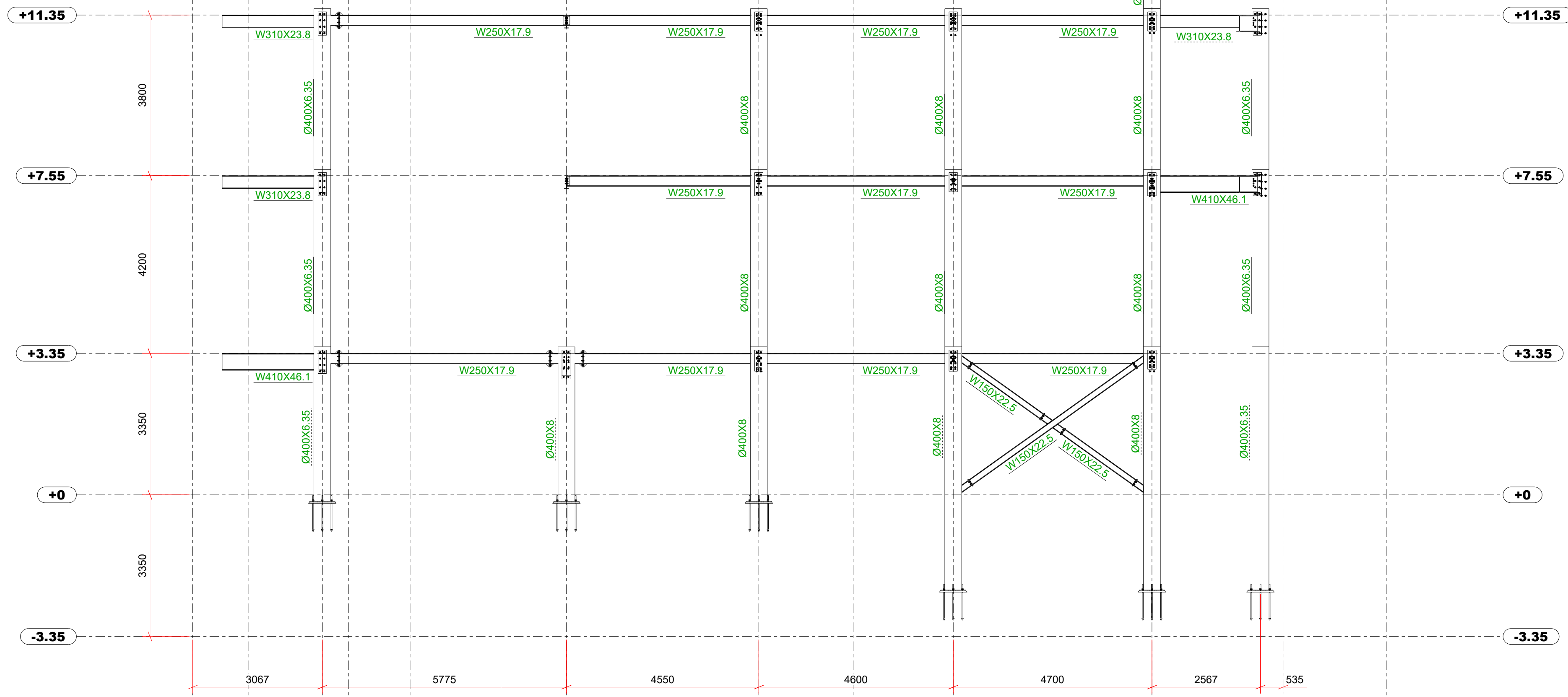
ELEVAÇÃO EIXO "12" ESC. 1:75
