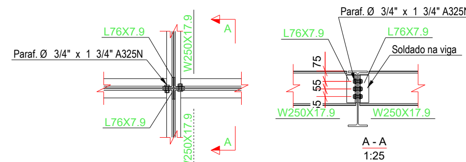
DET. TÍPICO W250 C/ VIGA
