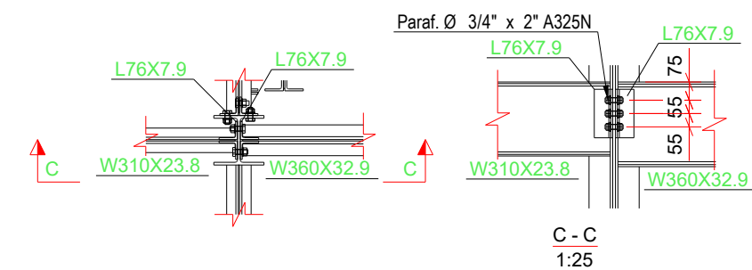
DET. TÍPICO W310 e W360
