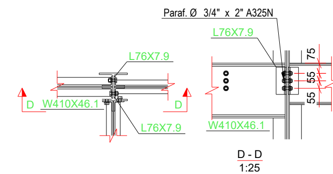
DET. TÍPICO W410
