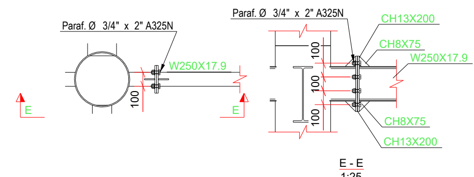
DET. TÍPICO W250 NO PILAR
