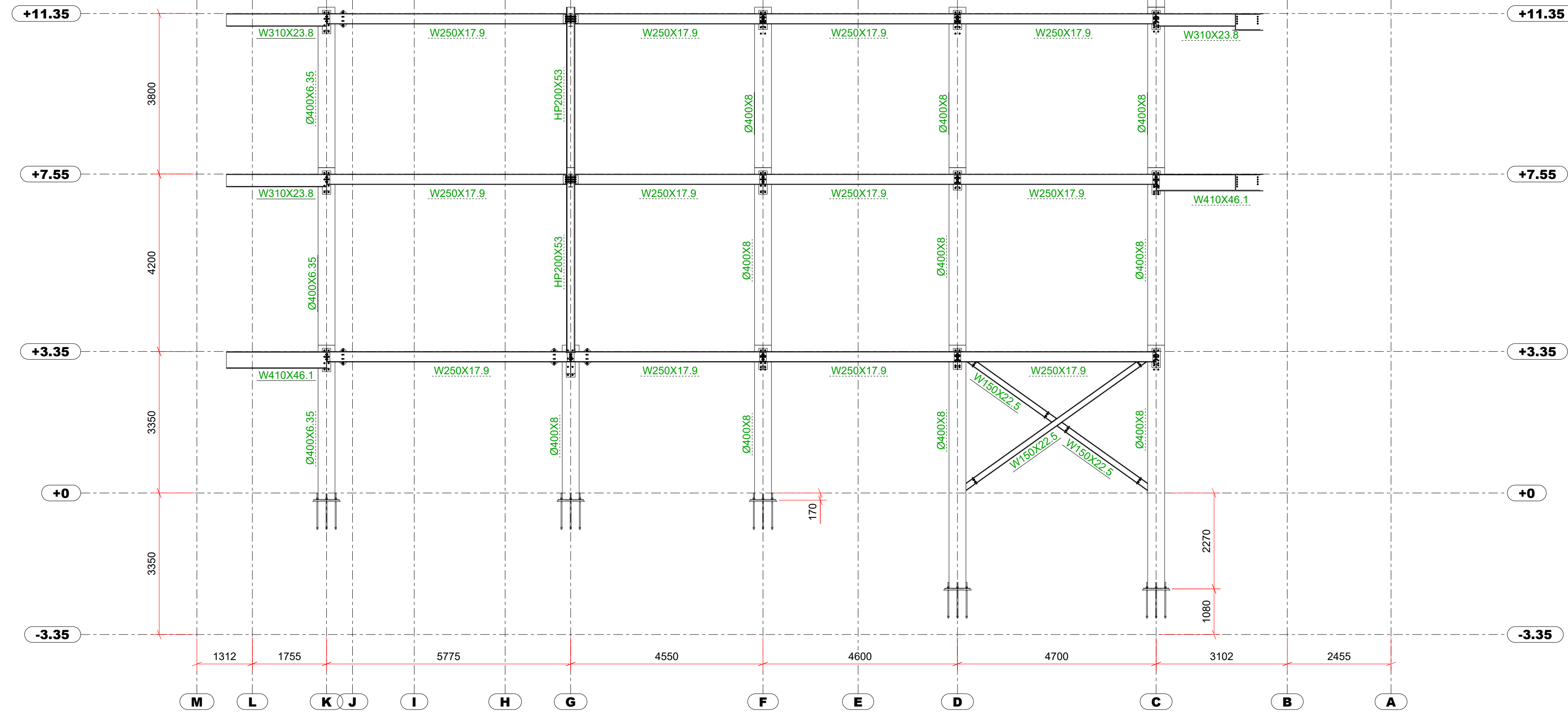
ELEVAÇÃO EIXO "11" ESC. 1:75
