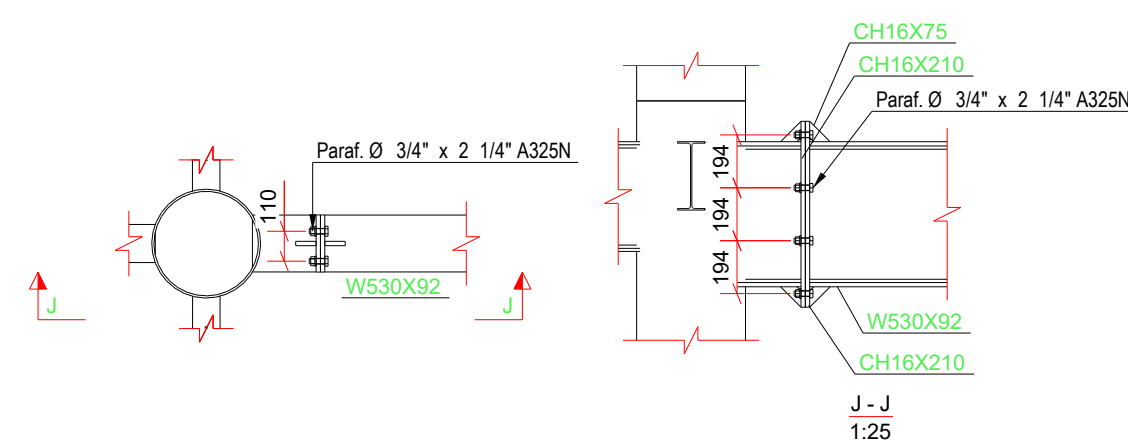
DET. TÍPICO W530 NO PILAR
