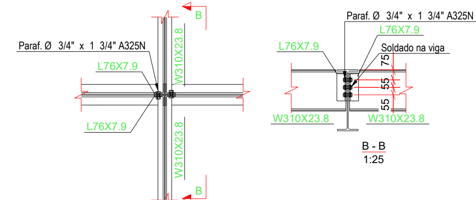
DET. TÍPICO W310 C/ VIGA
