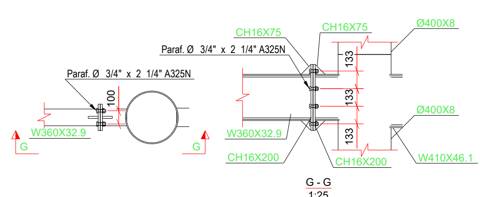
DET. TÍPICO W360 NO PILAR
