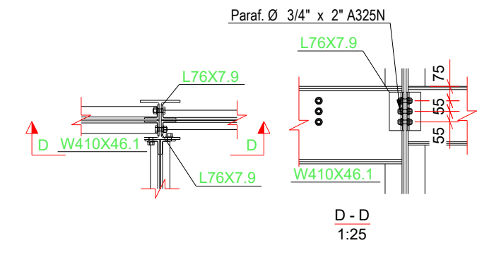
DET. TÍPICO W410
