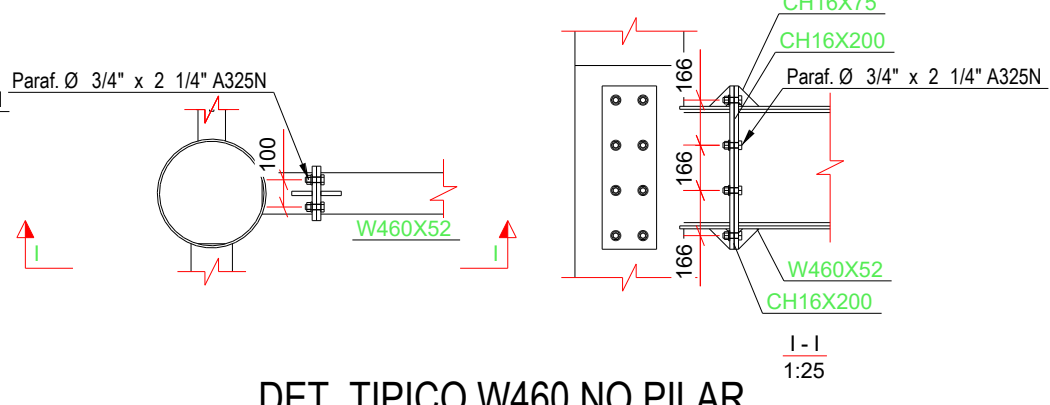
DET. TÍPICO W460 NO PILAR
