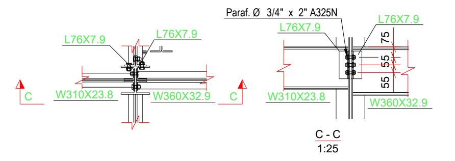
DET. TÍPICO W310 e W360
