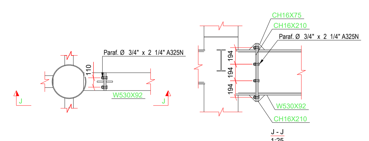
DET. TÍPICO W530 NO PILAR
