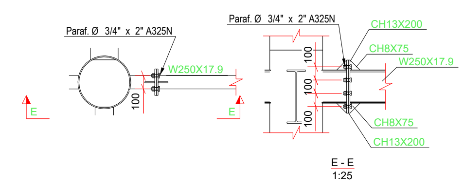
DET. TÍPICO W250 NO PILAR
