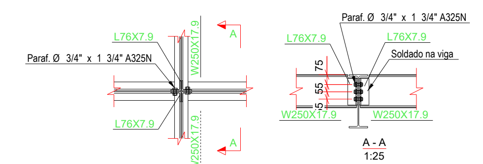
DET. TÍPICO W250 C/ VIGA
