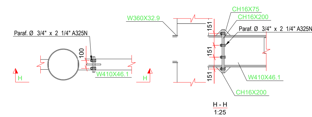
DET. TÍPICO W410 NO PILAR
