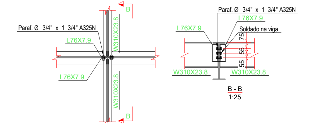
DET. TÍPICO W310 C/ VIGA
