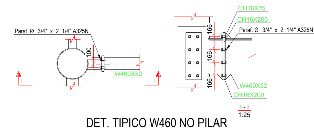
DET. TIPOCO W460 NO PILAR
