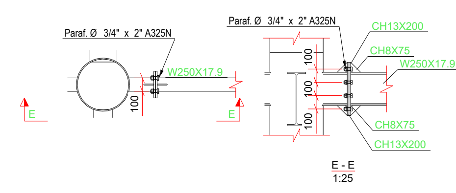
DET. TIPOCO W250 NO PILAR
