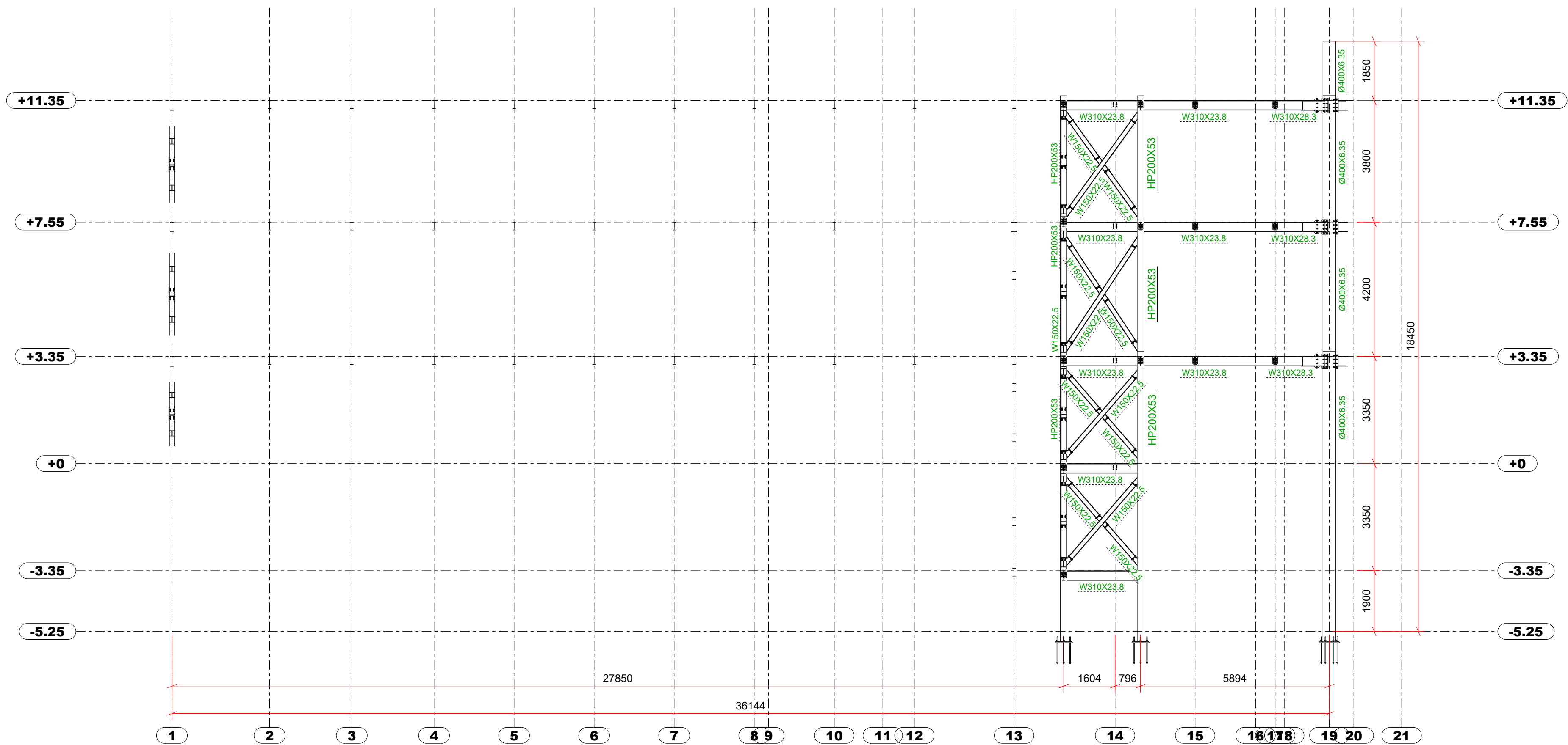
ELEVÇÃO FILA "I" ESC. 1:100
