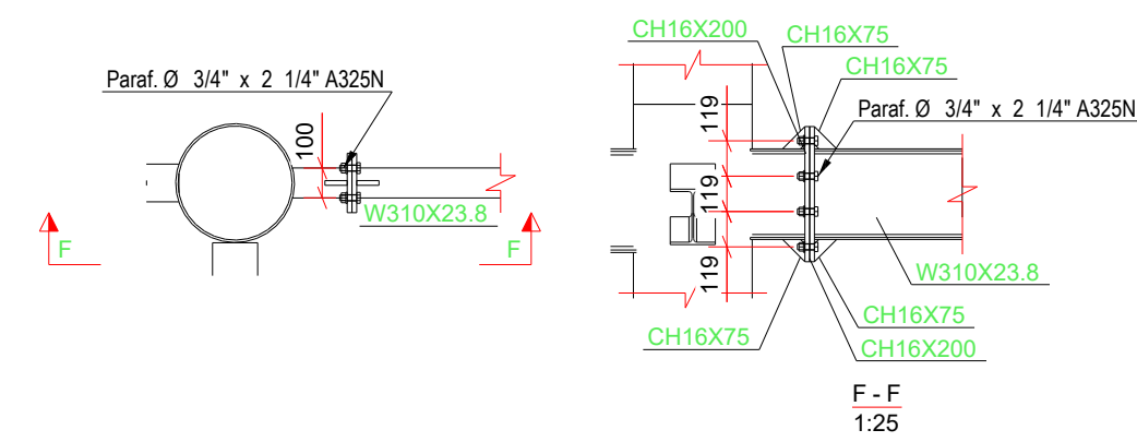
DET. TIPOCO W310 NO PILAR
