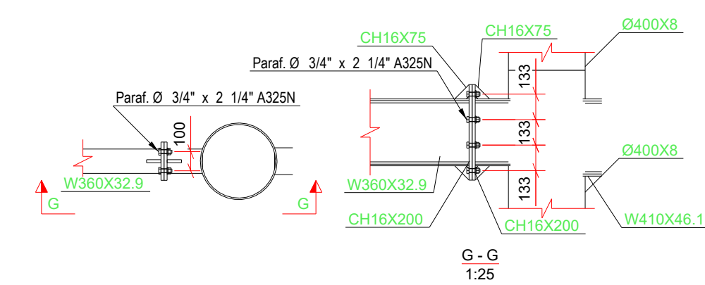
DET. TIPOCO W360 NO PILAR
