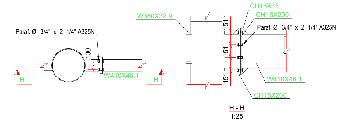
DET. TIPOCO W410 NO PILAR
