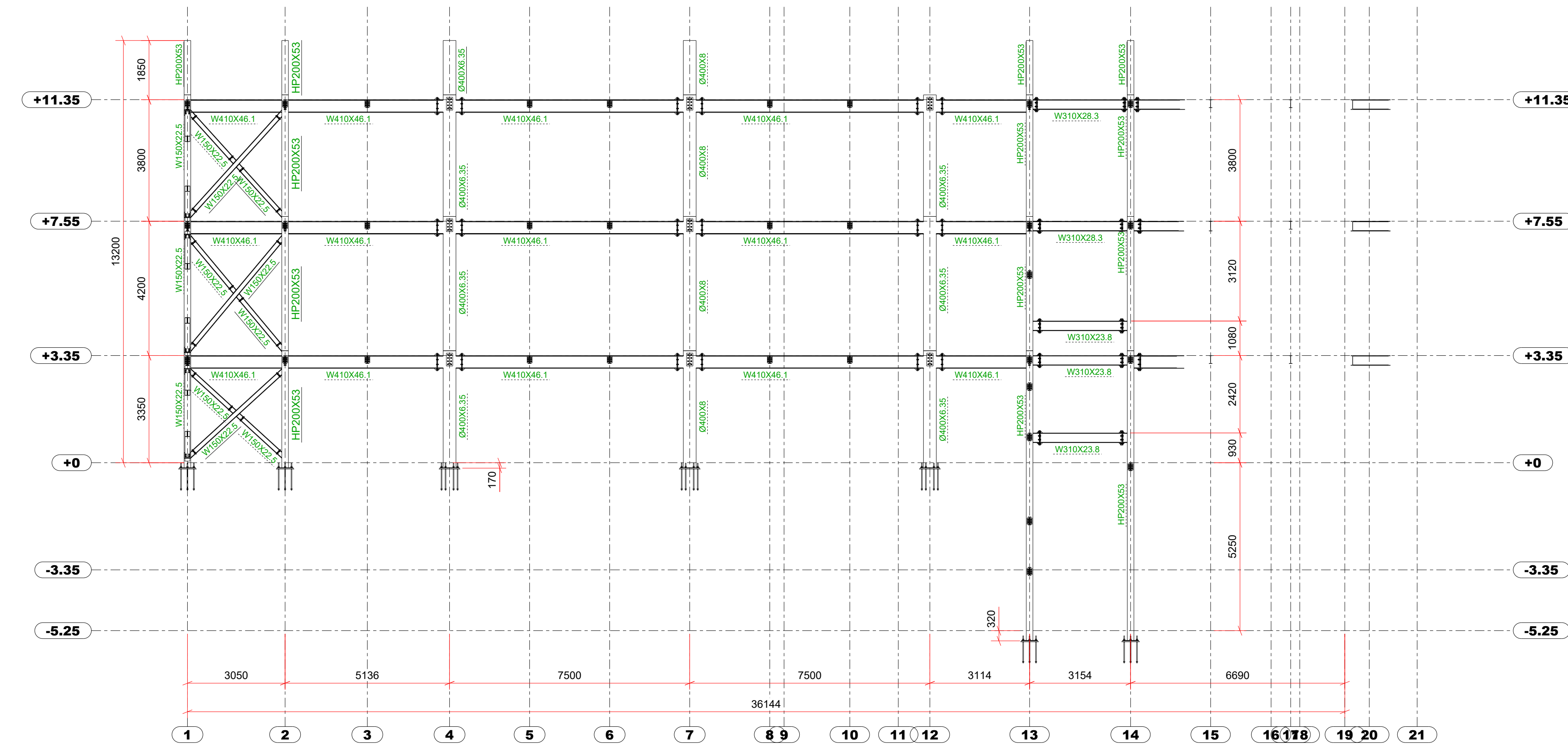
ELEVÇÃO FILA "J" ESC. 1:100
