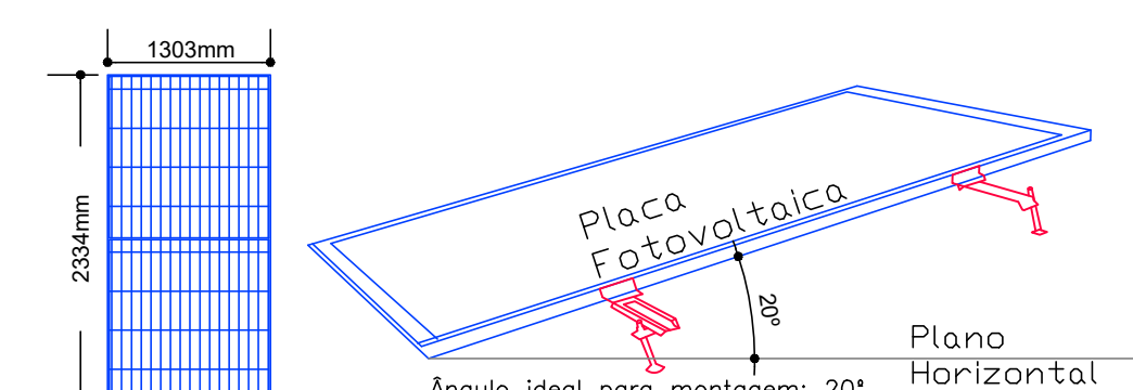
MONTAGEM DOS MÓDULOS SOLARES (TELHADO)
