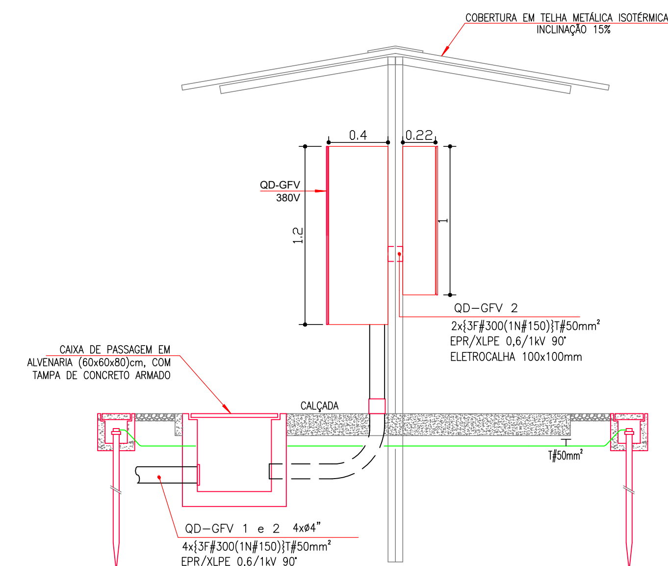
CORTE BB - ABRIGO DOS INVERSORES EXISTENTE ESCALA 1:25
