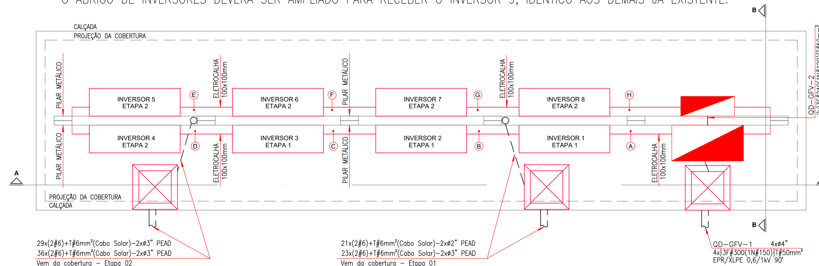
PLANTA BAIXA - ABRIGO DOS INVERSORES - EXISTENTE ESCALA 1:25
